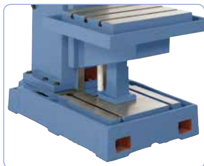
Masivní rozměrná základová deska s T-drážkami. Stůl lze demontovat - optimální k opravování vysokých obrobků. (z KBM 63).
