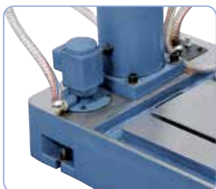
Čerpadlo chladicí kapaliny v základní výbavě
