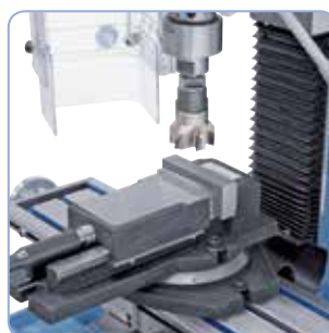
Frézování s plochou a rohovou frézou (pol. č.: 42-1058)
