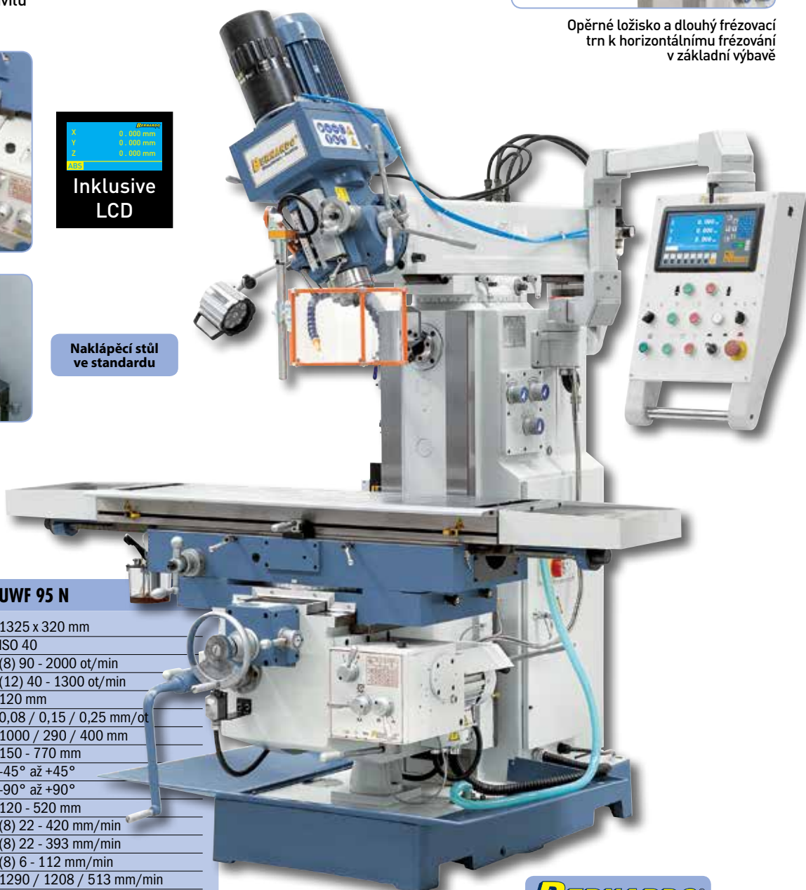
Masivní provedení vodících ploch v osách y, z zajišťuje zvýšenou stabilitu
