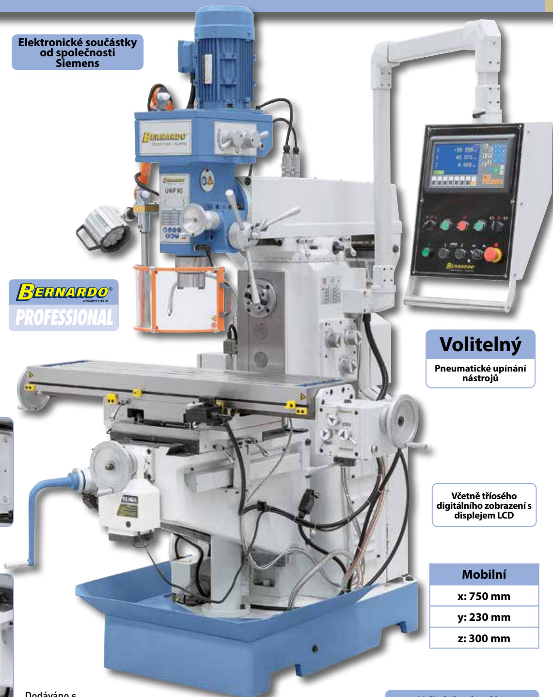
Jednoduché řazení převodů pohonu horizontálního vřetene v základní výbavě
