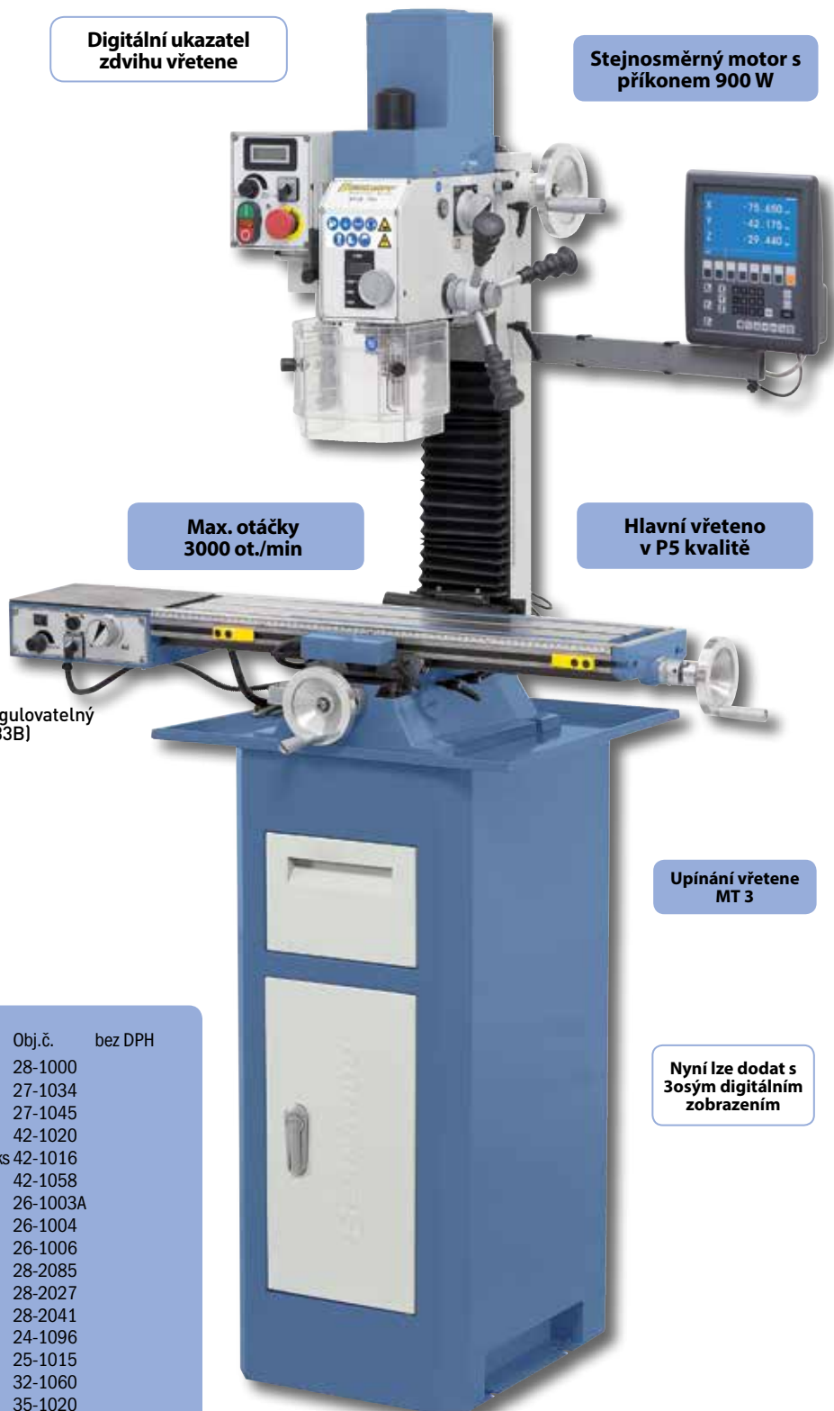
Digitální zobrazení Bernardo ES-12 V pro osu x a y je součástí dodávky (obj. č.: 02-1033B).
