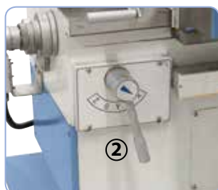
1. Páka pro směr posuvu 2. Páka pro osu posuvu
